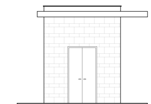
PROSPETTO OVEST
