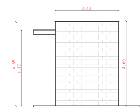
PROSPETTO EST
