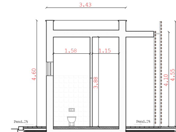
SEZIONE B-B'
