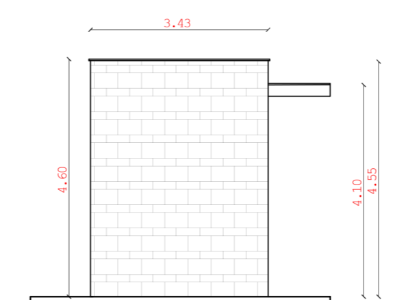
PROSPETTO OVEST
