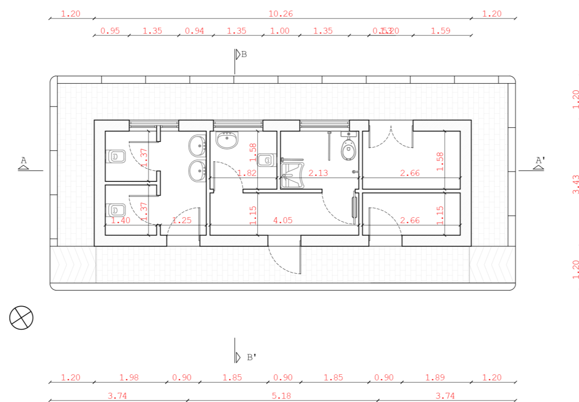
PLANIMETRIA
